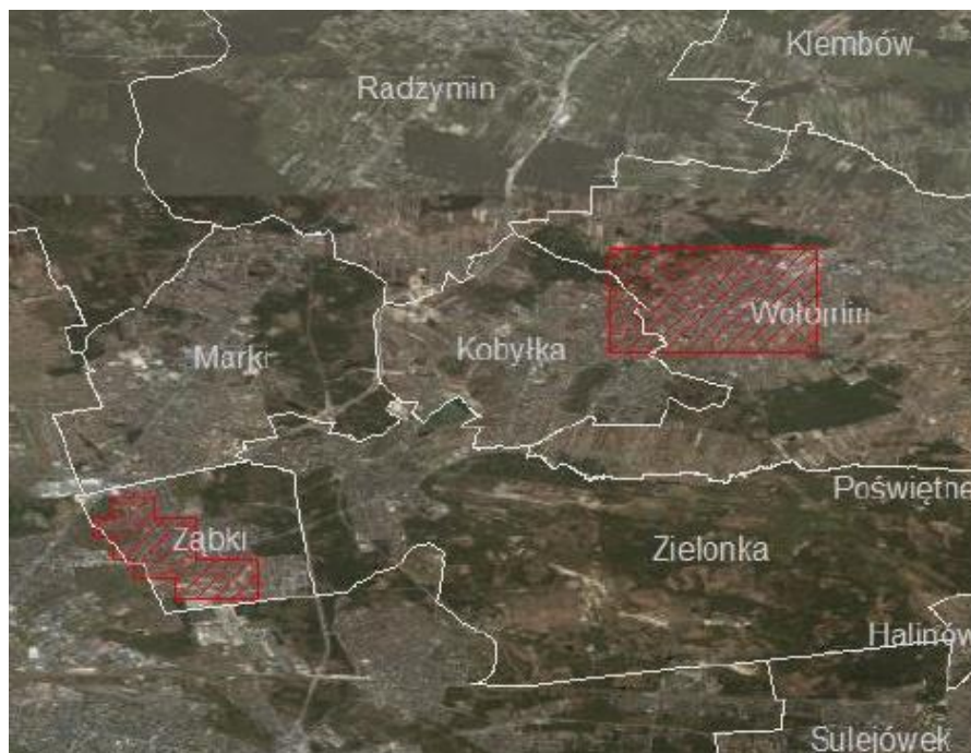
Rysunek 12. Obszary występowania przekroczeń stężenia pyłu zawieszonego PM 10 .
